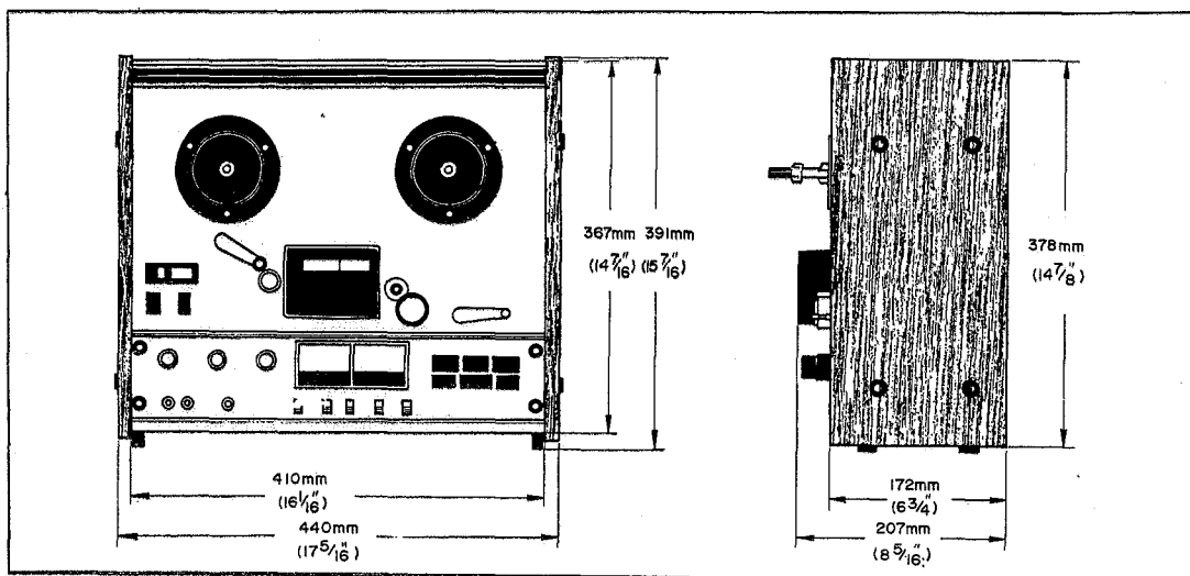
Fig. 2-2 Dimensions
